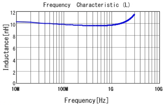
■ LQW15AN10NJ00 L
