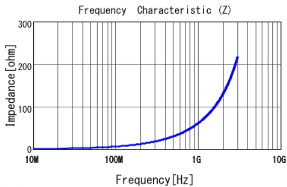
■ LQW15AN10NJ00 |Z|
