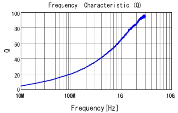
■ LQW15AN10NJ00 Q
