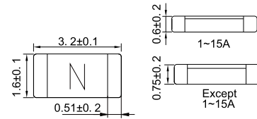
1206 Size
