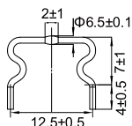
253 Size
