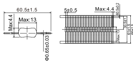
3.6x10 Size
