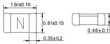
0603 Size
